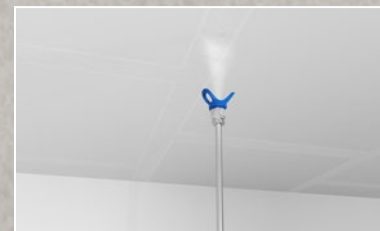
D / Ruiskuta vain saumat Ruiskuta yksi ohut kerros pintamassaa yhteen suuntaan vain saumoihin.
